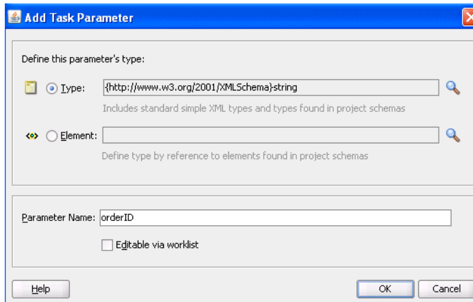
Figure 28–18 Add Task Parameter Dialog
