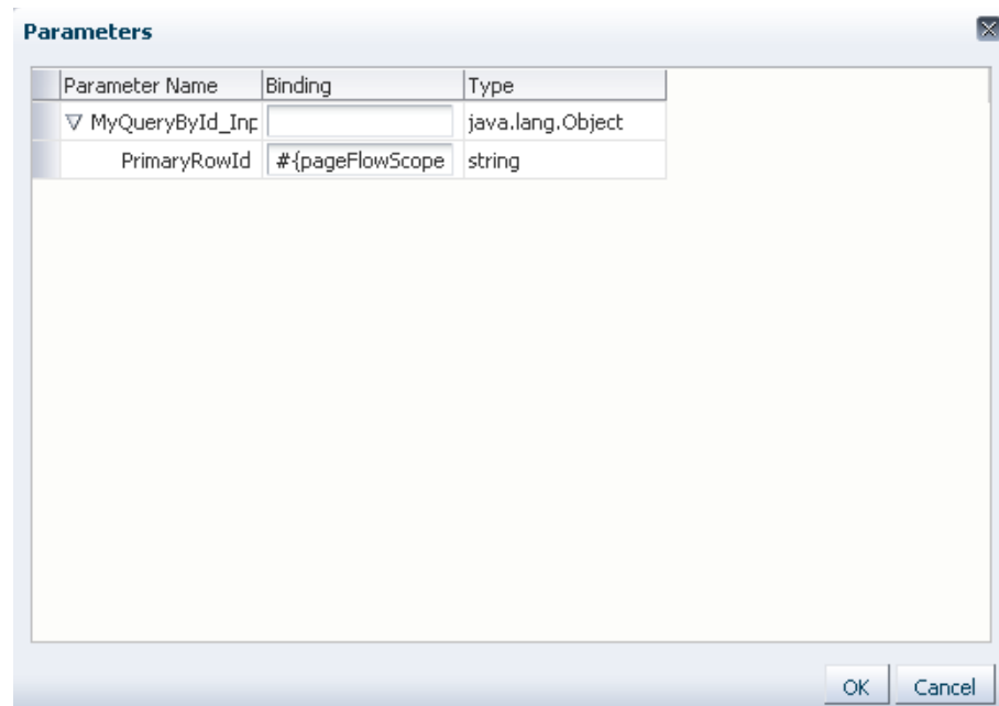
Figure C–26 Parameters Dialog
