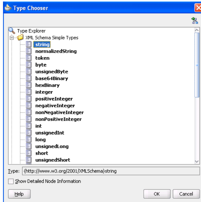
Figure 28–19 Parameter Type
